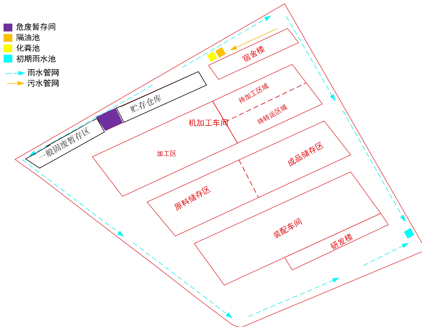
附图 4 项目雨污管网图
