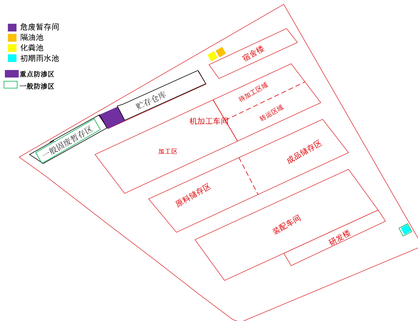
附图 3 项目厂区平面布置及分区防渗图
