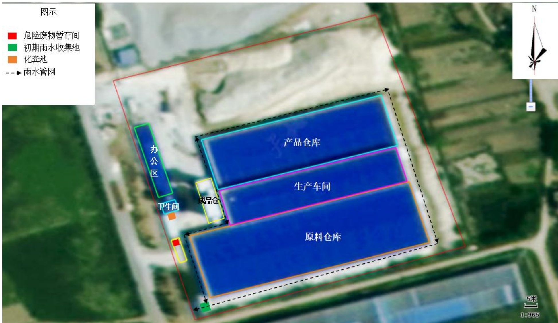
附图 5 雨污管网图
