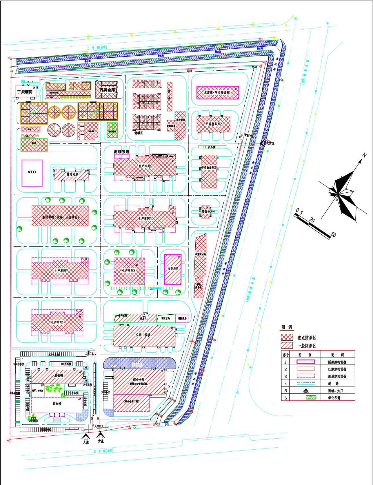
附图 5 项目厂区分区防渗图
